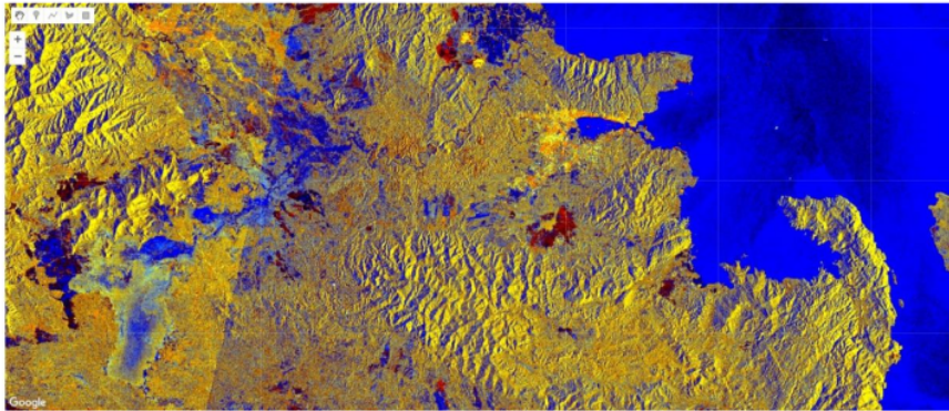
Gambar 3. Citra Satelit Sentinel 1 hasil pengolahan menggunakan GEE
