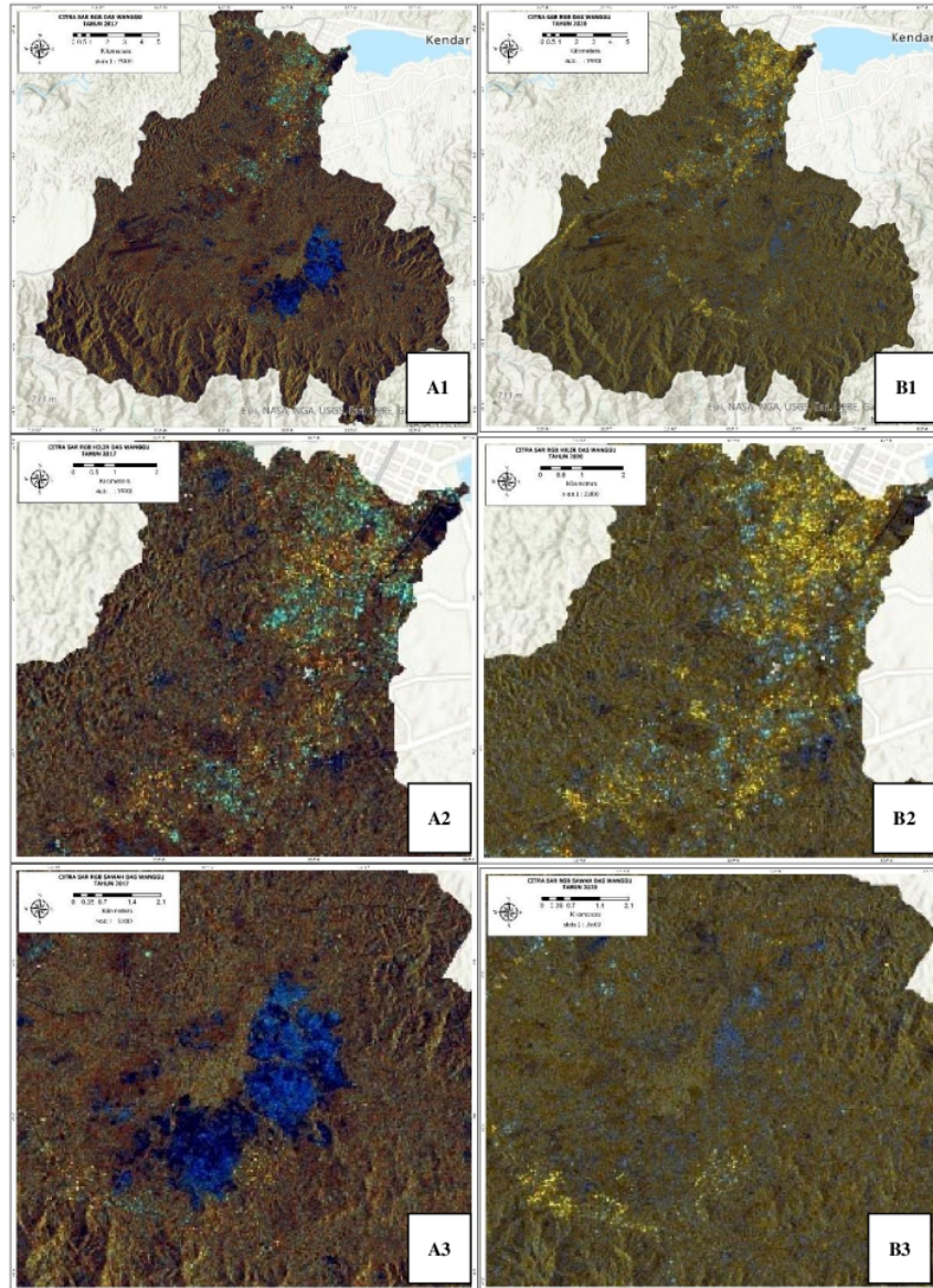
Gambar 4. Komposit RGB Sentinel 1 SAR pada DAS Wanggu
