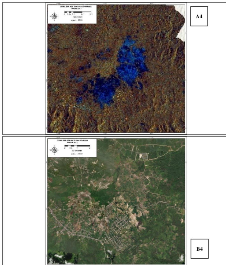
Gambar 5. Verifikasi hasil RGB SAR area persawahan
